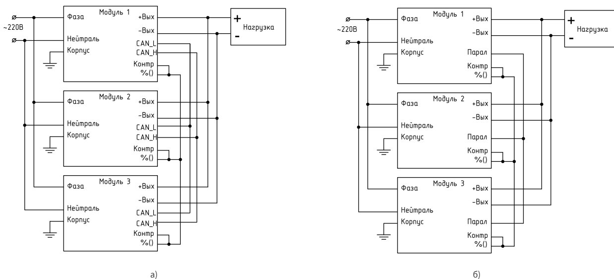
Рис.6.1а. Параллельное соединение КАН5000Ц30/60
